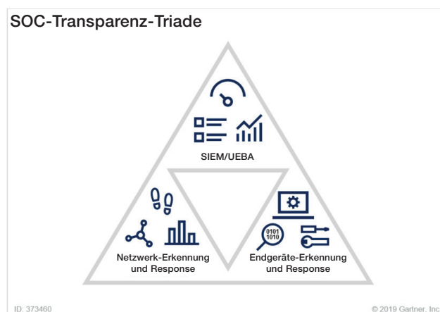
Abbildung 1. SOC-Transparenz-Triade
